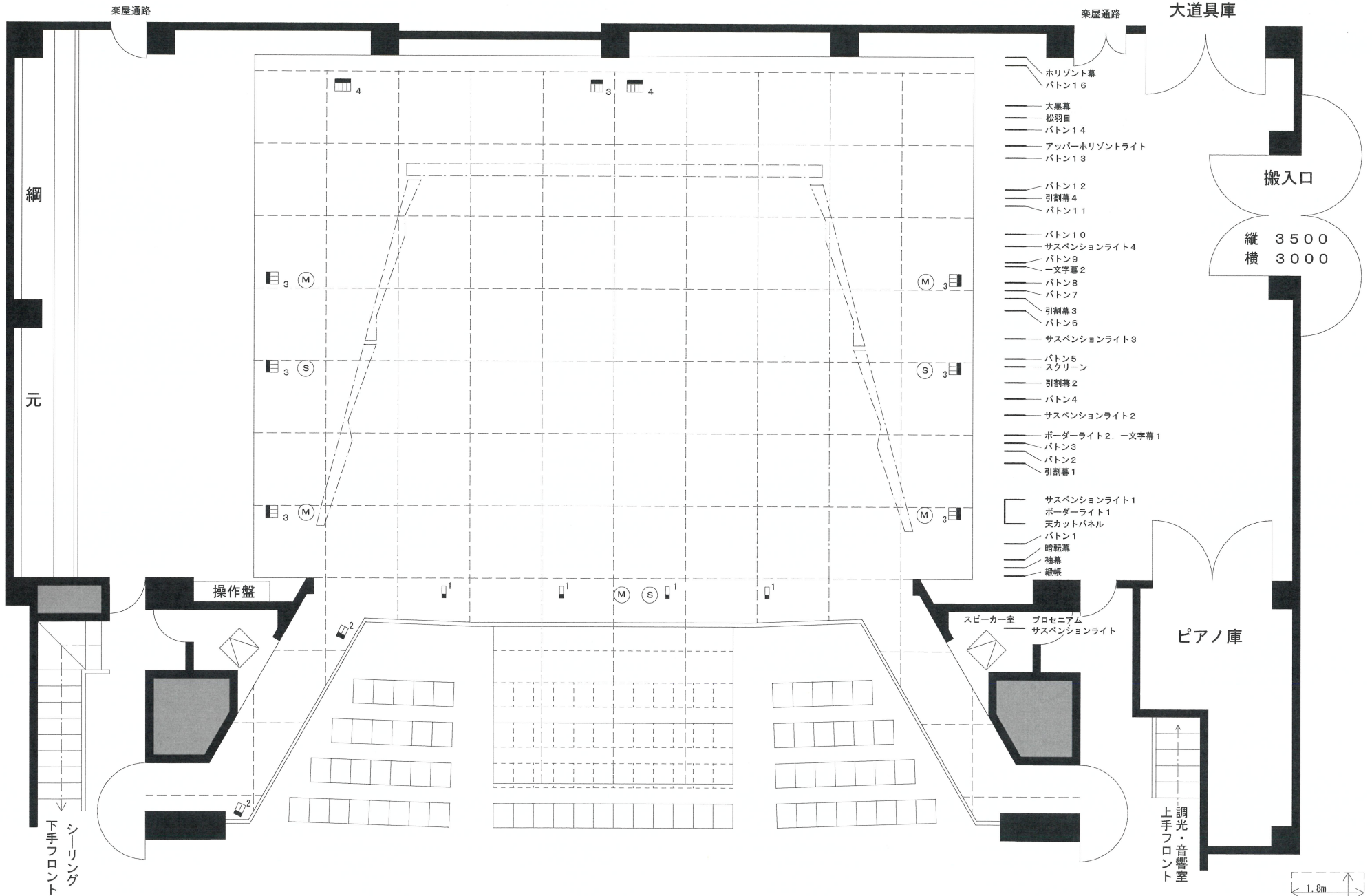
仙台市広瀬文化センター 舞台平面図 1/100
